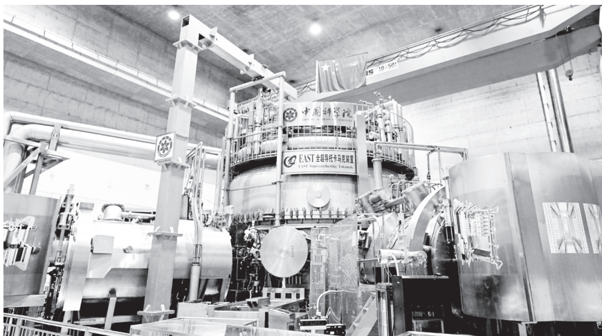
>> 2025年1月20日，中国有“人造太阳”之称的全超导托卡马克核聚变实验装置（EAST）在安徽合肥创造新的世界纪录，首次实现1亿摄氏度1066秒的高约束等离子体运行，标志我国聚变能源研究实现从基础科学向工程实践的重大跨越
